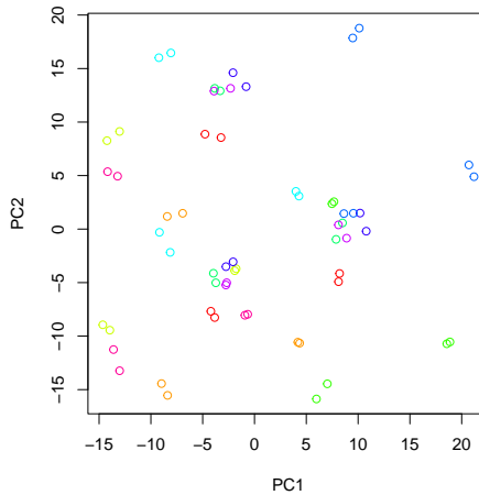
(d) hclust - colored by Individual
